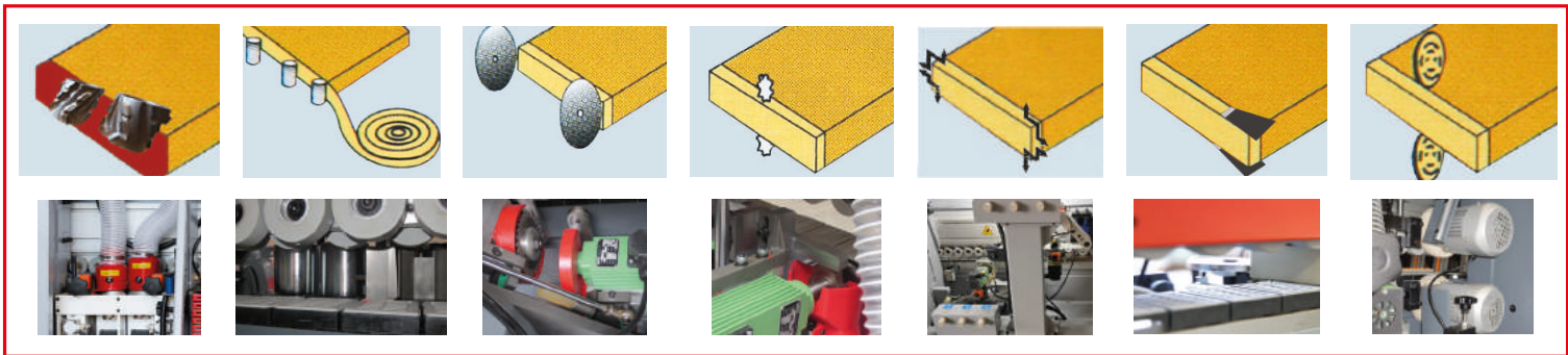
Vorfräser pre-milling
