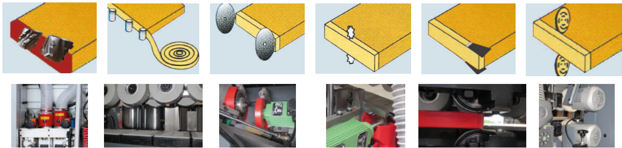
Vorfäser pre-milling
