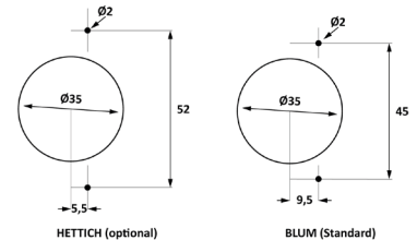
Hettich Wechselkopf hettich change head (optional)
