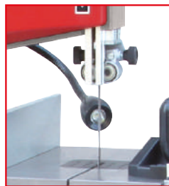
mit Halogenlampe with halogen lamp
